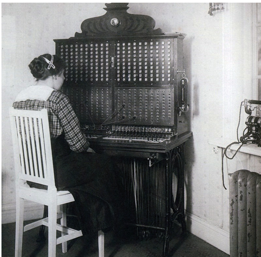
Ett exemplar av L M Ericssons 50-linjers telefonväxel från 1897, fotograferad ca 1915.
